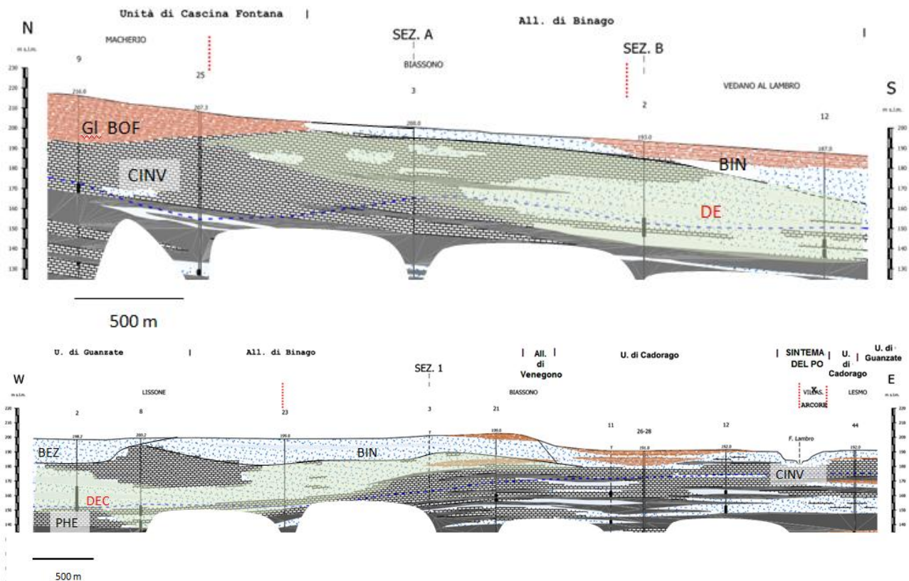
Figura 5: In alto rappresentazione del passaggio fra conglomerati e ghiaie alterate fra Macherio e Monza, tratta dai rilievi e dalle interessanti elaborazioni dello studio associato Boninsegni e Laveni sui Comuni della zona, fra i quali Biassono e Monza, che pone in luce la forte riduzione dello spessore totale del conglomerato fra Macherio e Vedano. La sigla DEC indica i terreni probabilmente soggetti a decementazione. In basso la sezione condotta al limite N del confine con Monza, evidenzia la riduzione dello spessore dei conglomerati procedendo verso Ovest. Il livello piezometrico si mantiene a profondità notevoli (decine di metri) dal piano campagna e l'acquifero saturo è costituito quasi esclusivamente da conglomerati.
