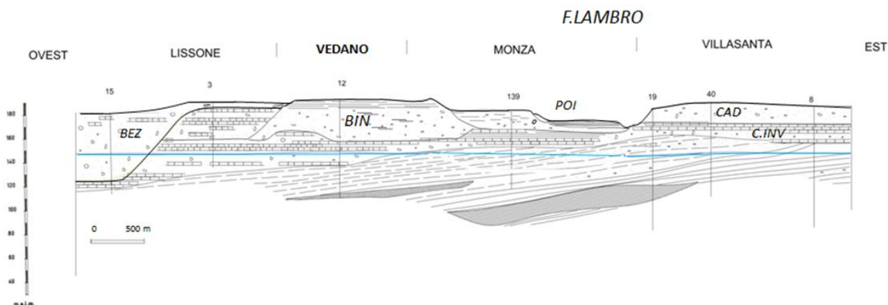
Figura 4: La sezione O-E fra Lissone e il Parco di Monza, poco a S della precedente, mostra la depressione del substrato colmata dai depositi del Paleo-Adda. Si nota la riduzione dello spessore complessivo dei conglomerati rispetto alla sezione passante O-E per Macherio (figura 4) che si trova a soli 2 km più a N e si ha conferma dello spessore complessivo dei conglomerati a Lissone. L'acquifero saturo è contenuto nei livelli cementati o nei livelli più superficiali dell'unità C.
