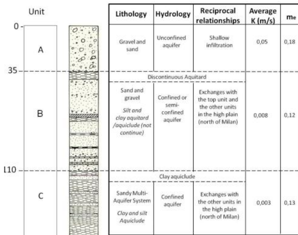
Figura 1 - Unità idrostratigrafiche dell'area milanese, secondo la classificazione ENI-Regione Lombardia, e loro parametri distintivi. Nello schema, che riporta i valori medi di questo parametri, vengono riportati anche informazioni sui possibili scambi idrici tra le unità (da V. Francani e al.)
