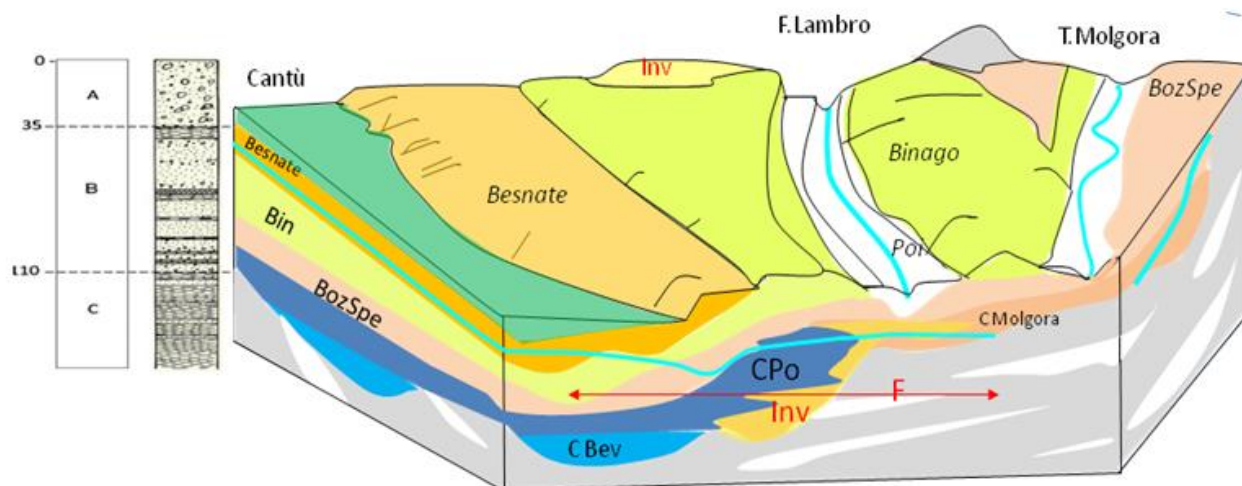
Figura 2: Lo schema evidenzia il fatto che nel Monzese, in prossimità del F. Lambro, l'acquifero è contenuto nelle unità ricche di conglomerati. In azzurro è rappresentato l'andamento del livello piezometrico e la morfologia piezometrica della depressione milanese (tratto F). E' indicato anche il possibile rapporto fra le unità idrostratigrafiche e quelle allostratigrafiche cartografate sul Foglio Seregno a scala 1/50.000., fra le attuali valli del F. Seveso e del t. Molgora. Con le sigle sono riportate le denominazioni delle diverse unità. Nella porzione occidentale dello schema si è ricordato l'avvallamento del substrato alla base dei conglomerati (porzione inferiore dell'unità B, figura 2) e la complessa morfologia del limite Binago-Besnate. In grigio è indicato il substrato costituito dalle alloformazioni Castel di Sotto e Lazzate, corrispondenti al Villafranchiano Auct. e all'unità idrostratigrafica C.
