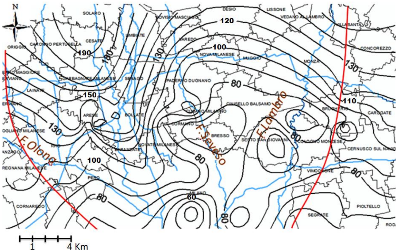
Figura 3: linee di livello del tetto del substrato (unità C) nell'area di studio. Si nota l'avvallamento approssimativamente coincidente con la valle attuale del f. Seveso fra Cesano Maderno, Desio, Monza, Sesto SG, colmato in prevalenza dai conglomerati della base dell'unità B. Al limite Ovest della figura appare un tratto dell'avvallamento del substrato coincidente con la valle del F. Olona privo di conglomerati e con acquiferi di rilevante spessore. Sono indicati i limiti della depressione piezometrica che attualmente insiste su Milano, Sesto e Monza, che vengono a saldarsi poco a valle del centro storico di Milano.
